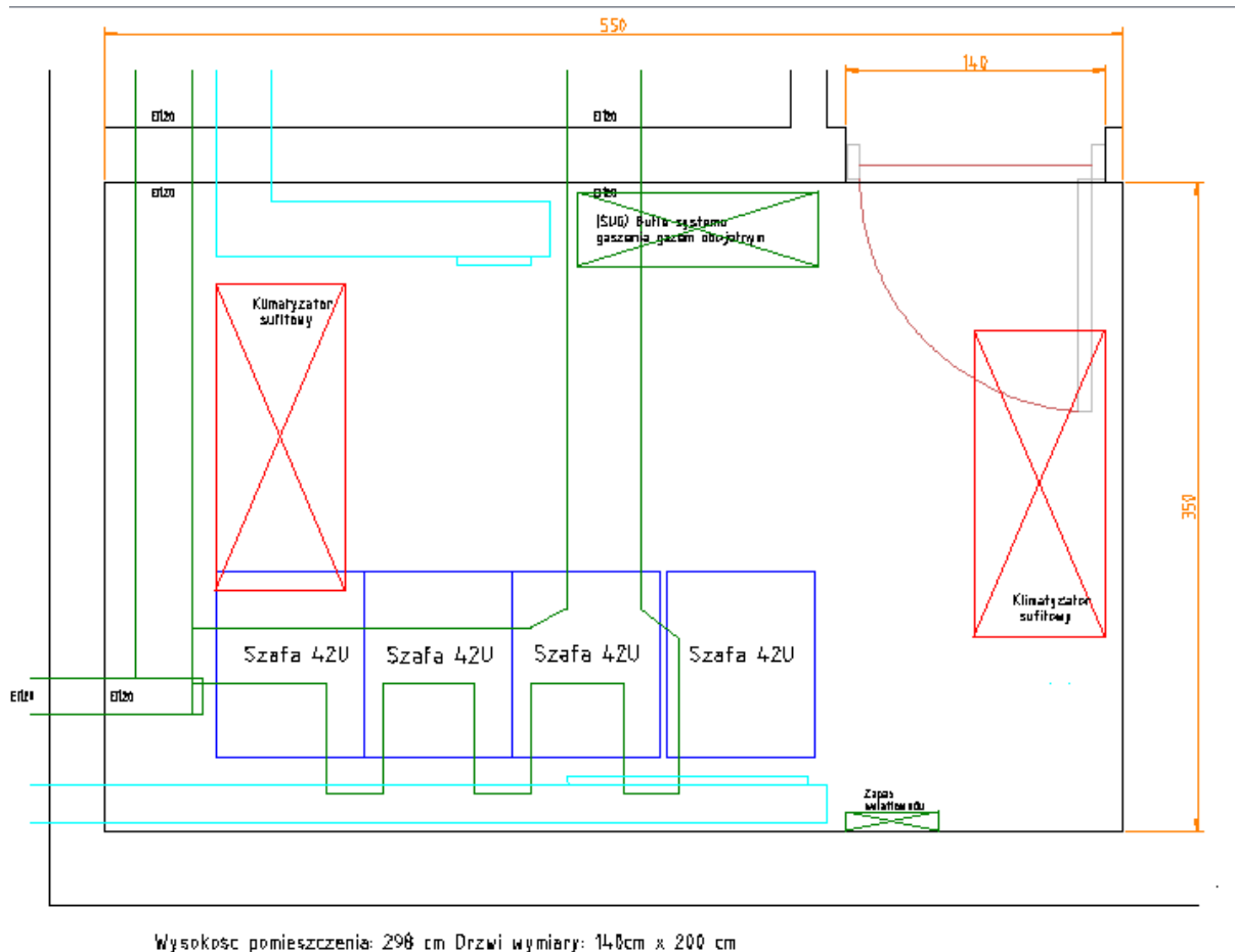
Rys. Proponowane rozmieszczenie serwerowni 2
