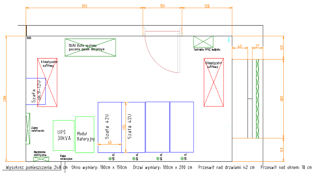
Rys. Proponowane rozmieszczenie serwerowni 1
